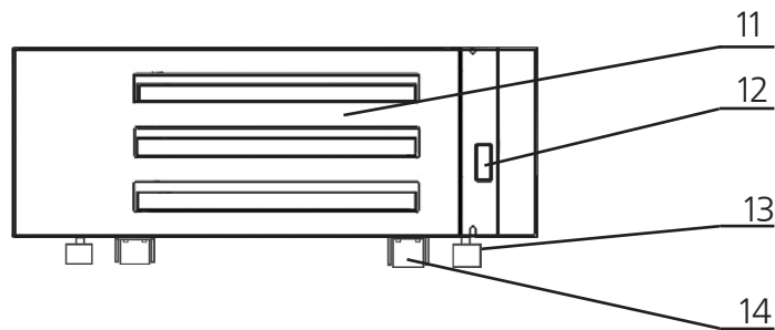
11 - облицовочная панель; 12 - автомат аварийного выключения шкафа; 13 - опора; 14 - ролик
